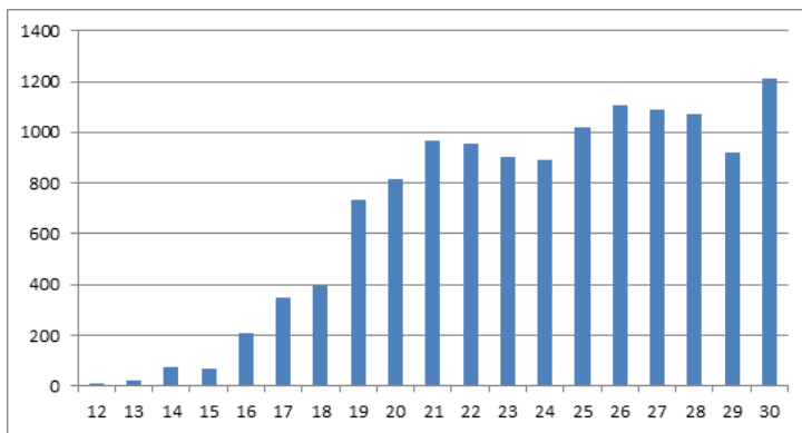
GRÁFICO 3 - Número de óbitos no Brasil, média diária por semana epidemiológica
