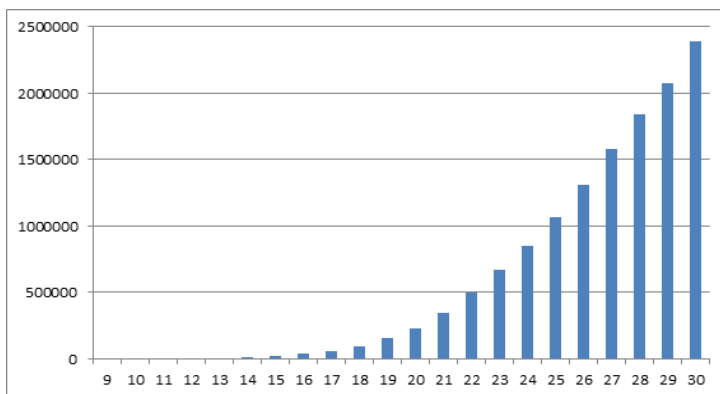
GRÁFICO 1 - Casos acumulados de covid-19 no Brasil, por semana epidemiológica
