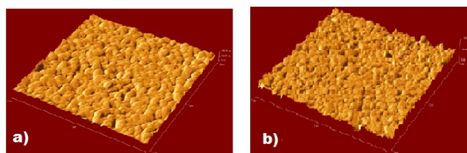
Figura 2. Imagens do ouro funcionalizado feitas pelo AFM a) filme octanotiol rugosidade média 2,0017nm; b) filme de 3-MPA, rugosidade média 2,3934nm.
