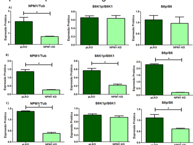
Figura 1. Knockdown de NPM1 em células HEK293, PC3 e DU145 diminui a fosforilação de S6Ks. A)-C) Gráficos mostrando a diferença estatística na expressão de NPM1 e fosforilação de S6K1 e S6 em HEK293, PC3 e DU145 respectivamente. Usado teste t de Student com n = 3 . * p < 0,05 .
