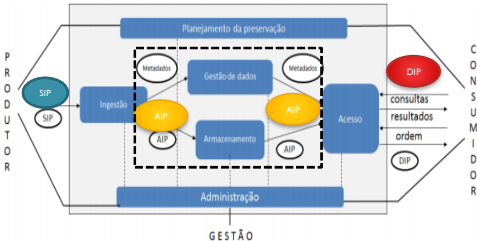
Figura 1. Modelo OAIS para preservação digital
